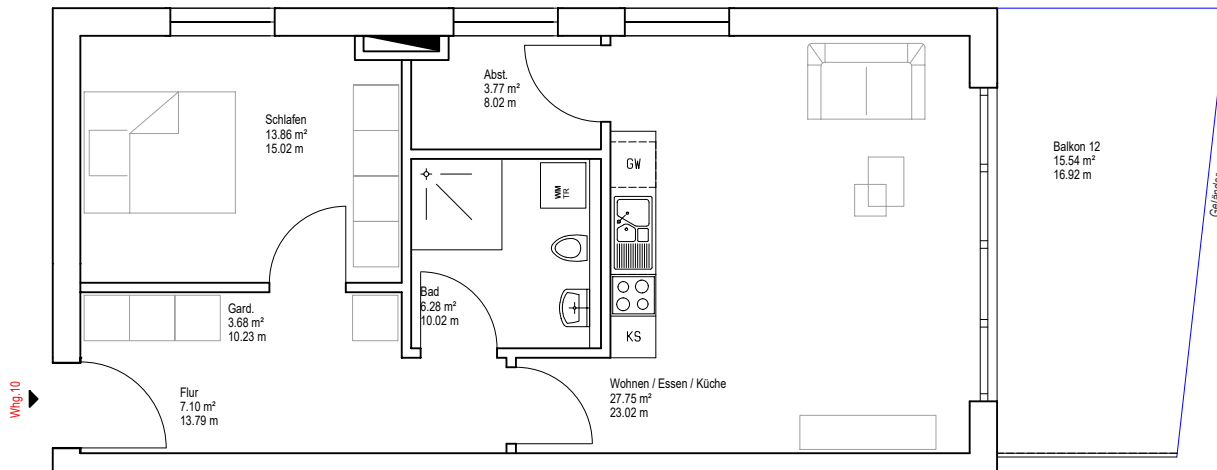
Musterwohnung 10 HH 1. OG M 1:100
