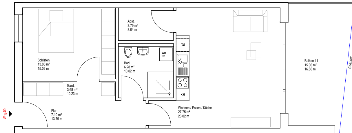
Musterwohnung 09 HH 1. OG M 1:100
